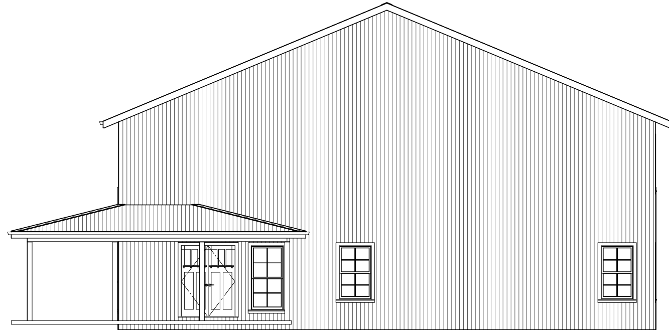
Right Elevation
