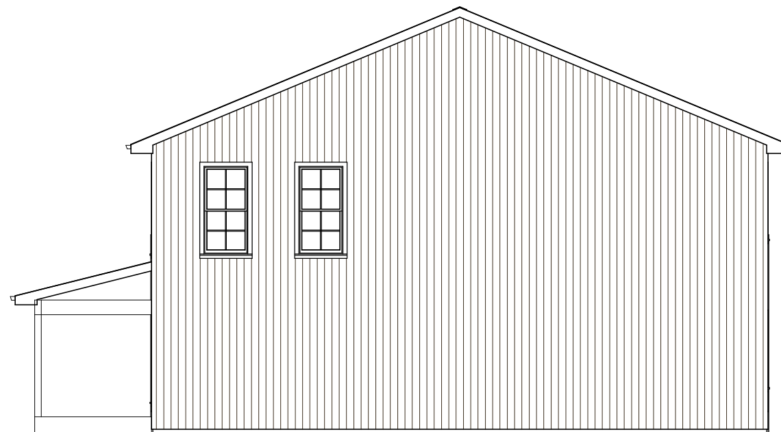
Right Elevation
